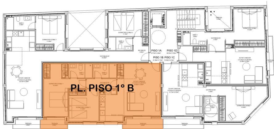
SITUACION VIVIENDA PLANTA PISO 1º
